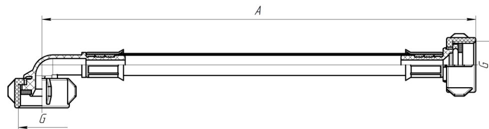
Рисунок 2 – Габаритные и присоединительные размеры изделия
