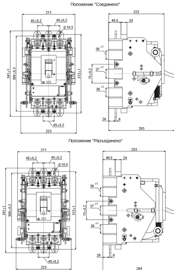
Рисунок 7 – Габаритные, установочные и присоединительные размеры выключателей выдвижного исполнения
