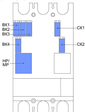
Рисунок 9 – Схема расположения гнезд под вспомогательные контакты, независимый или минимальный расцепители
