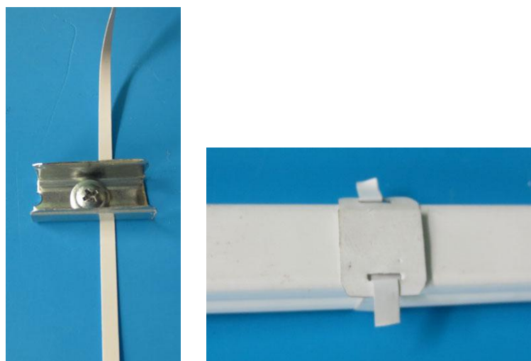
Рис. 23. Фиксация полупрофильного кабель-канала (верх).
