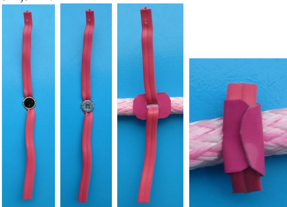
Рис. 9. Порядок установки дюбель–хомута КФСТ.735322.049.
