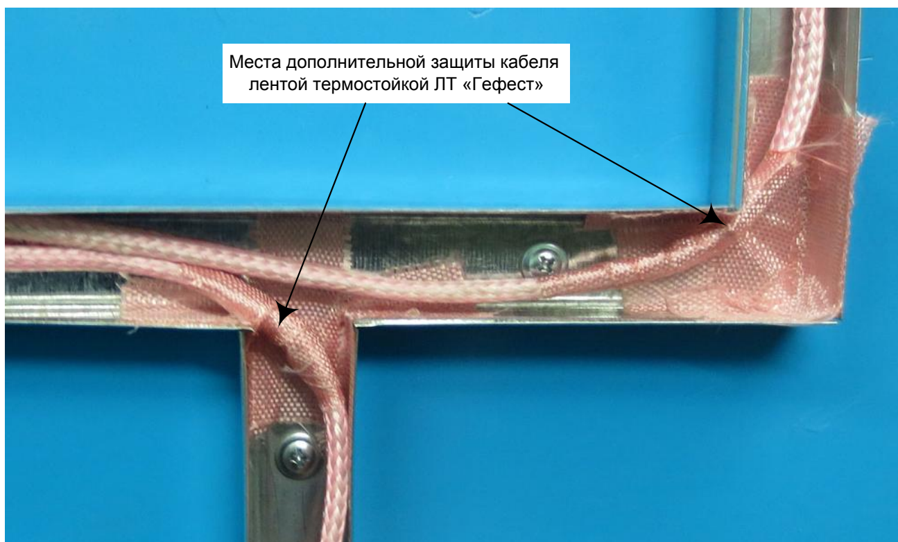
Рис. 20. Укладка КГО «Саламандра» в ККМО.
