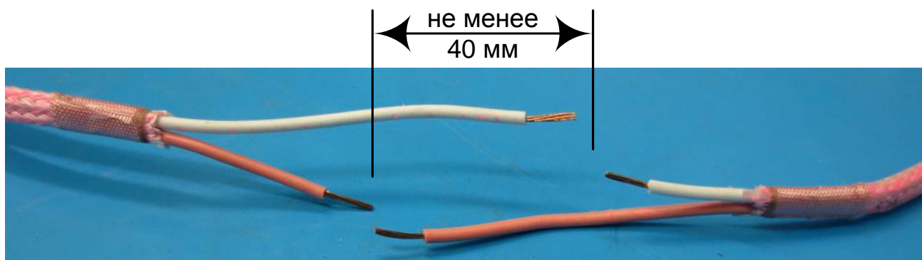
Рис. 28. Разделка кабелей для наращивания.
