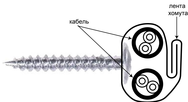
Рис. 7. Установка дюбель–хомута КФСТ.735322.041. Вариант 3.
