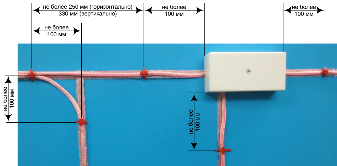
Рис. 16. Открытая прокладка кабеля по ленте основания.
