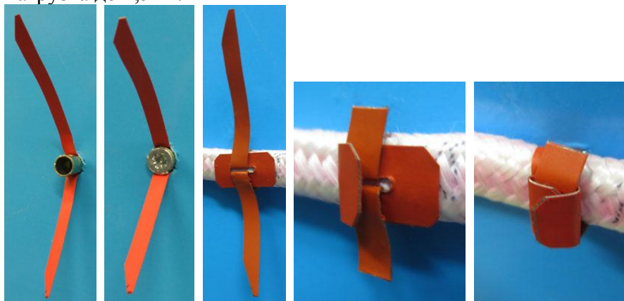
Рис. 11. Порядок установки дюбель–хомута КФСТ.735322.049-01.
