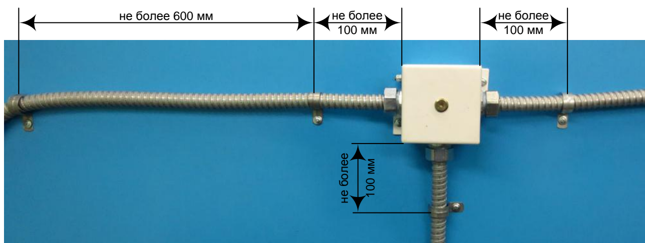
Рис. 17. Прокладка КЛ в металлическом рукаве.
