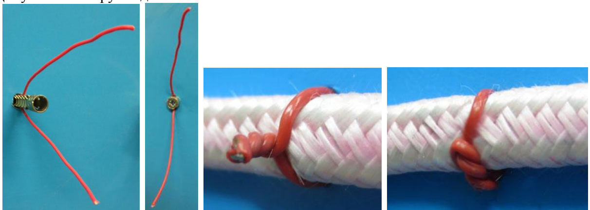
Рис. 13. Порядок установки дюбель–хомута КФСТ.735322.049-02.
