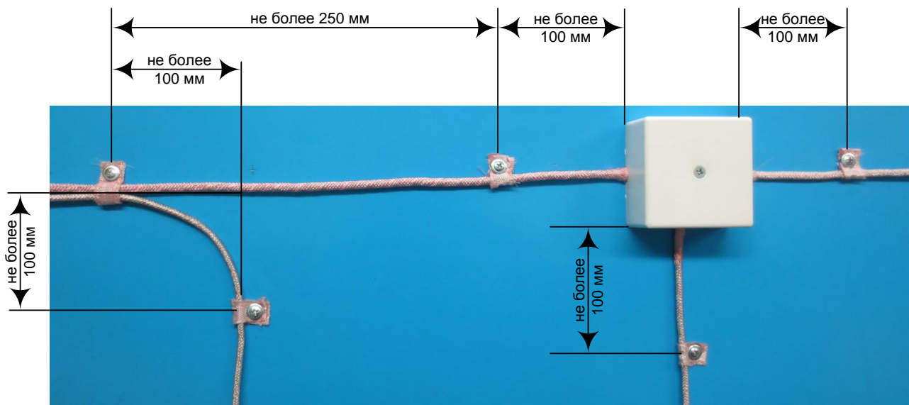
Рис. 14. Открытая прокладка кабеля.
