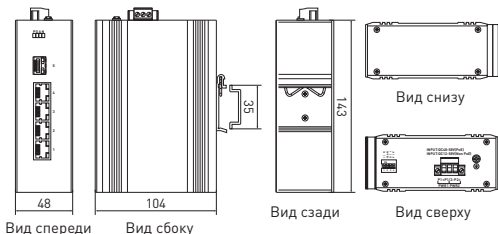
Рис. 1 — Габаритные размеры TSX-U-1GX/SFP-4GTP
