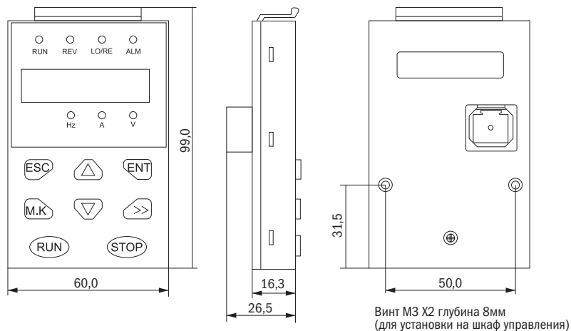
Схема 3.1.6 – Размеры пульта управления (мм)
