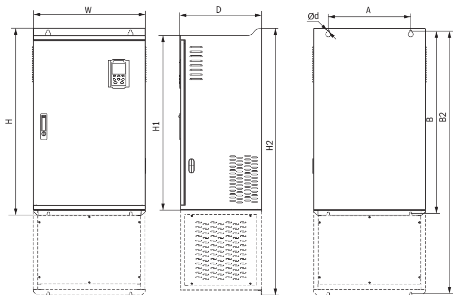
Рисунок 3.1.11 – Габаритные и установочные размеры габаритов 7+10 (110+250 кВт)
