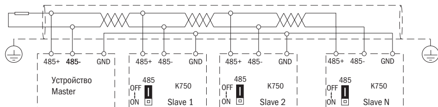
Рисунок 3.2.14 – Подключение нескольких преобразователей K750 в промышленную сеть с управлением от внешнего ПЛК
