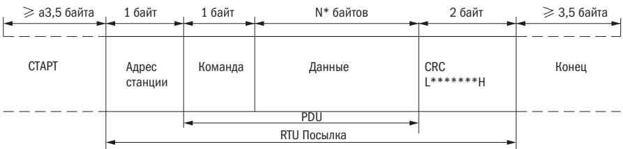
Рисунок А.1 – Структура посылки по протоколу MODBUS
