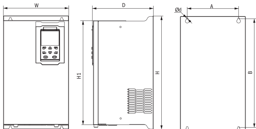
Рисунок 3.1.10 – Габаритные и установочные размеры габаритов 3+6 (18,5+90 кВт)
