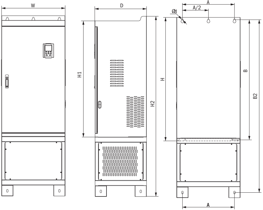
Рисунок 3.1.12 – Габаритные и установочные размеры габарита 11 (280+315 кВт)
