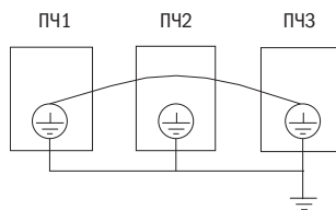
Рисунок 3.2.15 – Схема заземления преобразователей частоты
