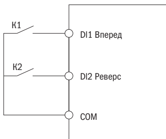
2-проводной режим 1
