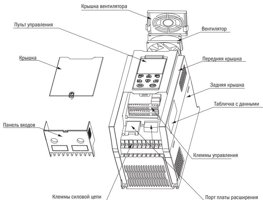
Рисунок 3.1.1 – Внешний вид преобразователей мощностью 0,75÷15 кВт
