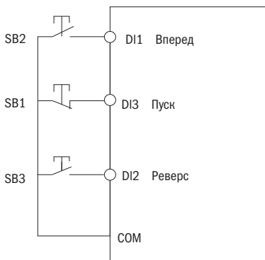
3-проводной режим 1
