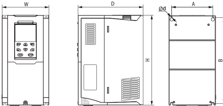
Рисунок 3.1.9 – Габаритные и установочные размеры габаритов 1+2 (5,5+15 кВт)
