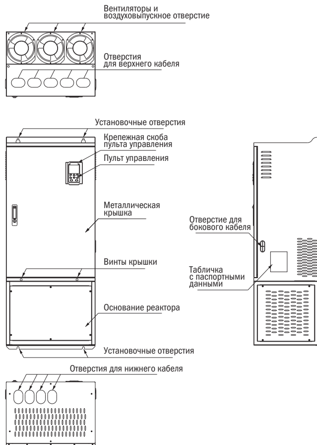
Рисунок 3.1.4 – Внешний вид преобразователей мощностью 110+250 кВт (с нижним основанием)
