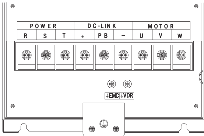
Рисунок 3.2.4 – Клеммы силовой цепи габарита 4 (30÷37 кВт)
