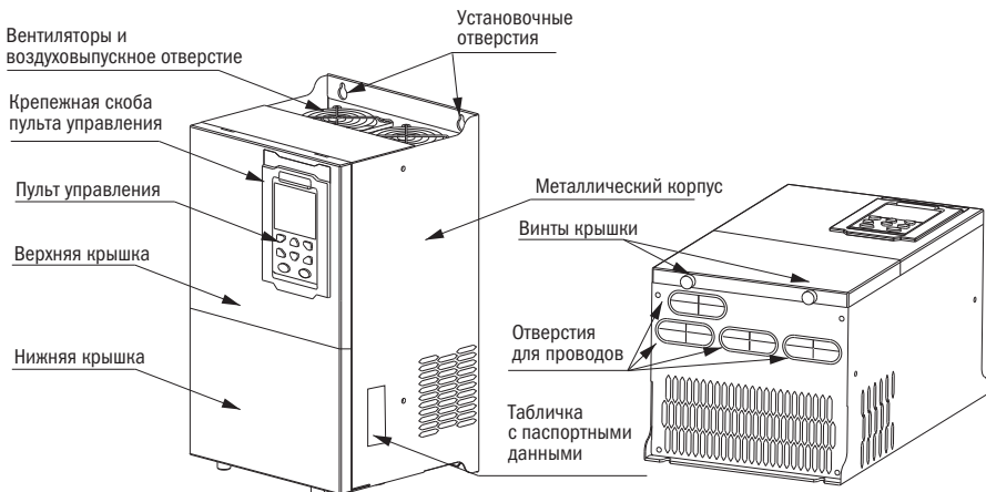
Рисунок 3.1.2 – Внешний вид преобразователей мощностью 18,5+90 кВт
