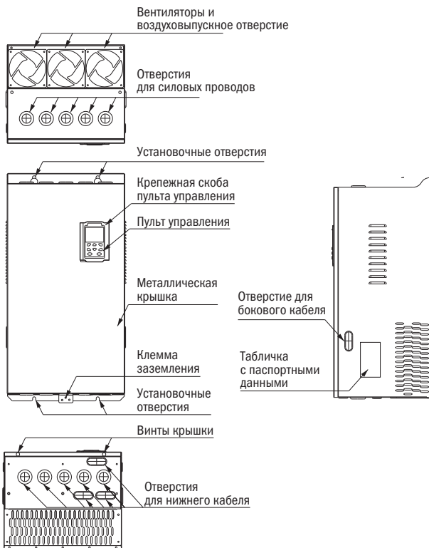
Рисунок 3.1.3 – Внешний вид преобразователей мощностью 110+250 кВт
