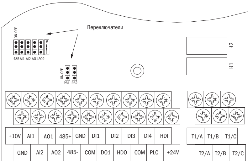
Рисунок 3.2.8 – Расположение клемм платы управления K750
