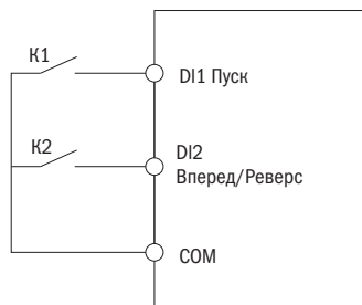
2-проводной режим 2
