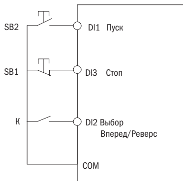
3-проводной режим 2
