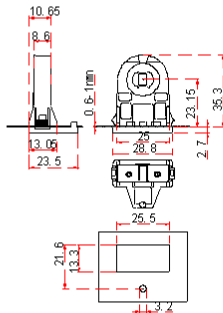
Патрон (ламподержатель) G13 для сквозного крепления с тыльной стороны, h- оси 23mm, со стопором, для T8, T12 люминесцентных ламп (крепление на боковые защелки)
