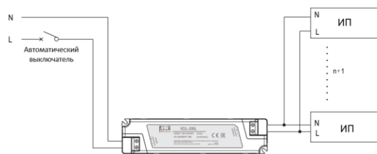
Схема подключения ICL-16L
