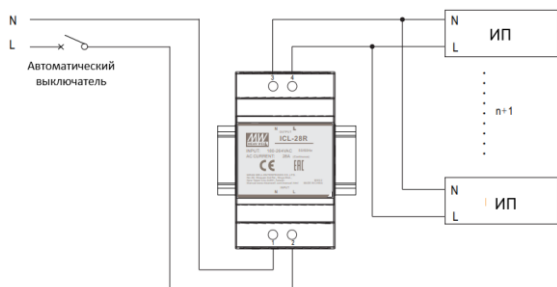
Схема подключения ICL-16R
