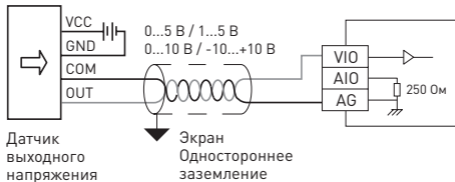
Рис. 4b - Подключение аналоговых входов (входной сигнал – напряжение)
