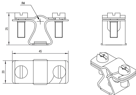
Рисунок 1 – Габаритные размеры
