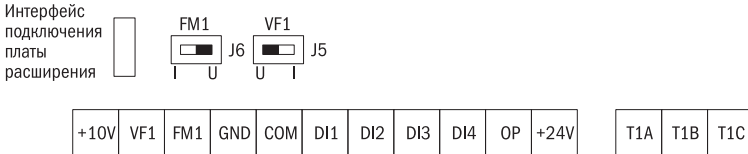
Рисунок 12 – Клеммная колодка платы управления преобразователя
