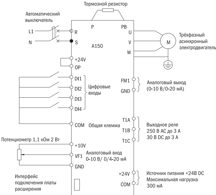
Рисунок 12 – Клеммная колодка платы управления преобразователя
