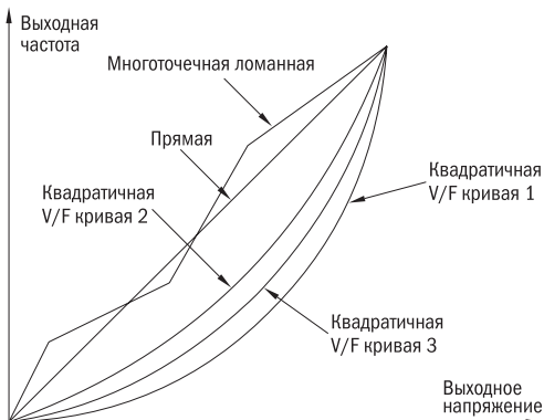
Рисунок 29 – V/F-кривые
