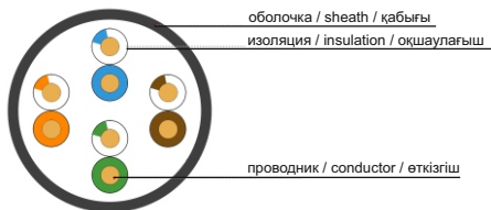
Рисунок 2 – Конструкция кабеля типа U/UTP (число жил 4x2) /
