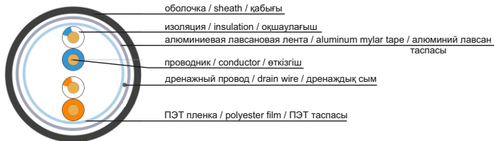
Рисунок 3 – Конструкция кабеля типа F/UTP (число жил 2x2) /
