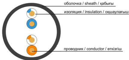
Рисунок 1 – Конструкция кабеля типа U/UTP (количество жил 2x2) / Figure 1 – Cable design of U/UTP type (number of cores 2x2) / Сурет 1 – U/UTP типті кабель дизайны (2x2 талсымдар саны)
