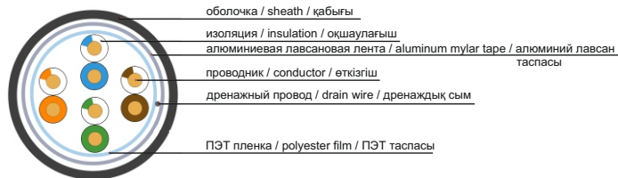
Рисунок 4 – Конструкция кабеля типа F/UTP (число жил 4x2) /
