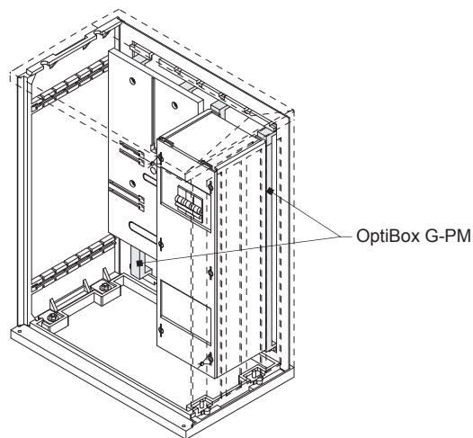
OptiBox G-PM
